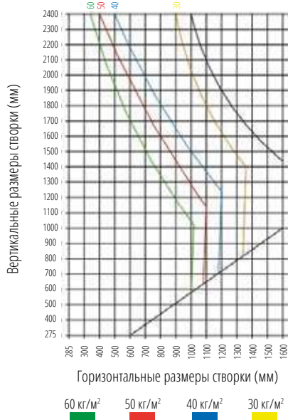
Диаграмма максимальных размеров створки допустимый вес створки 80 кг
