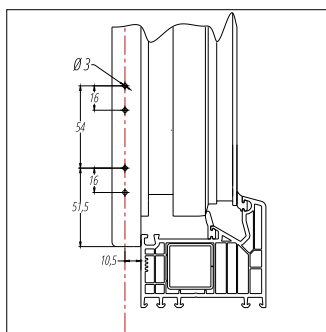
ПЕТЛЯ НИЖНЯЯ СТВОРКИ 80 КГ
