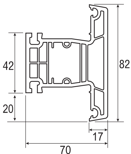
3.1.3 Профиль импоста арт. 7531M
