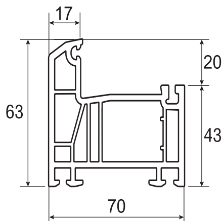
3.1.1 Профиль рамы арт. 7511M
