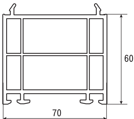
3.1.10 Профиль расширительный 60 мм арт. БР 362
