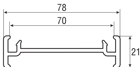
3.1.7 Профиль соединительный арт. БД 350
