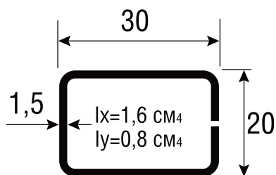
5.1 Армирующий профиль арт. 203 для арт. 5831M4K, 506, БР1144, 7531M, 385.06, 360
