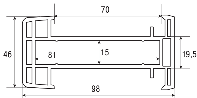
3.1.15 Н-образный соединитель арт. БД 352/118
