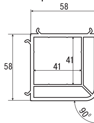
2.1.10 Угловой соединитель арт. 612
