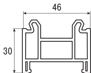
3.1.6 Профиль подставочный арт. 342
