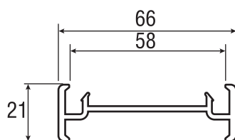
2.1.9 Профиль соединительный арт. БД 150
