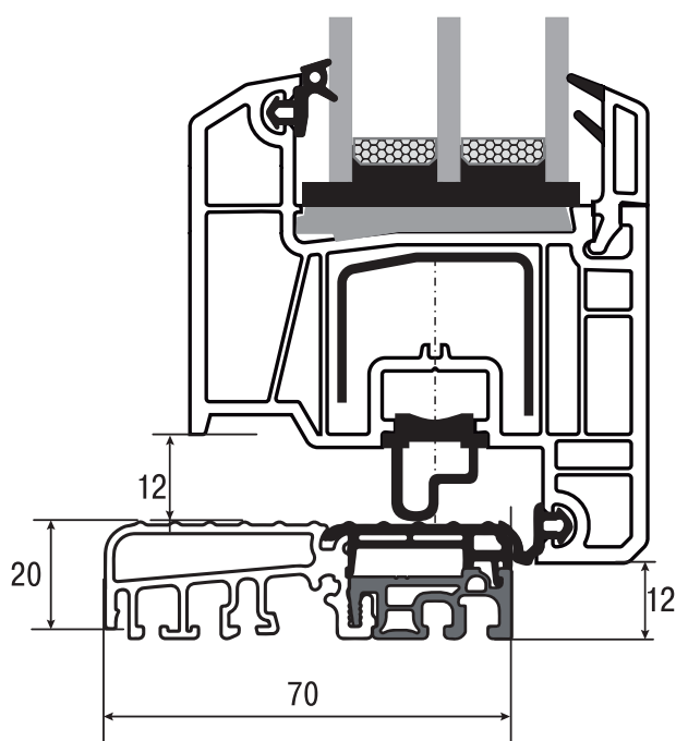
4.3 Система 7500 с теплым порогом
