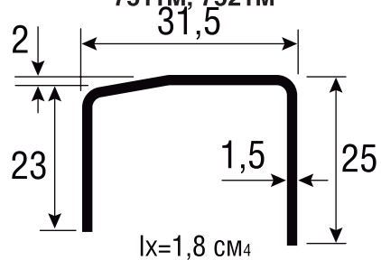
5.2 Армирующий профиль арт. 207 для арт. 5811M4K, 5821M4K, 7511M, 7521M
