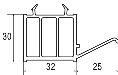
2.1.7 Профиль подставочный арт. 343 с крылом
