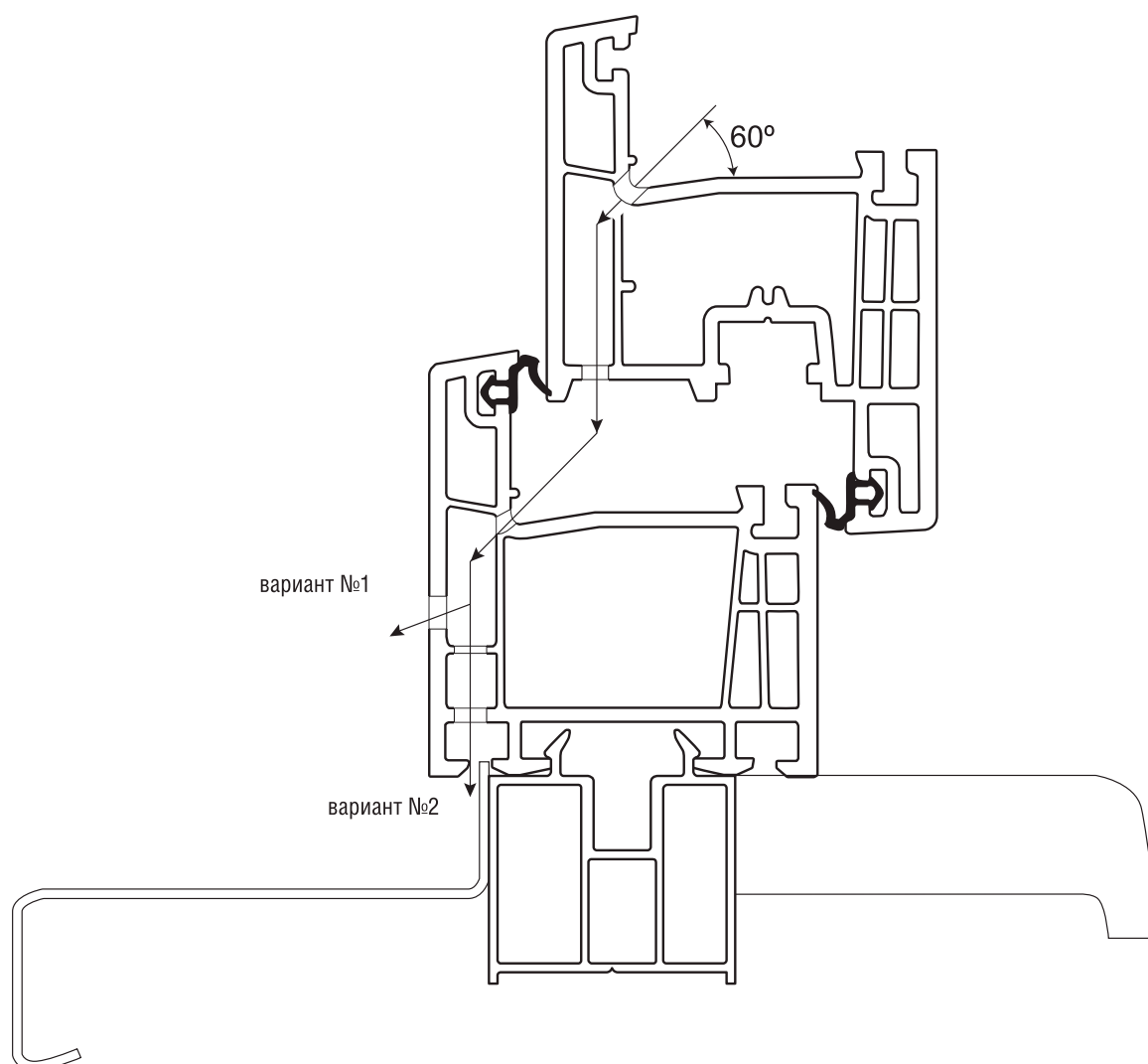
Схема водоотвода в раме и створке
