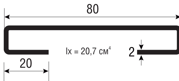
5.4 Армирующий профиль арт. 208, для арт.018/152, БД 352/118
