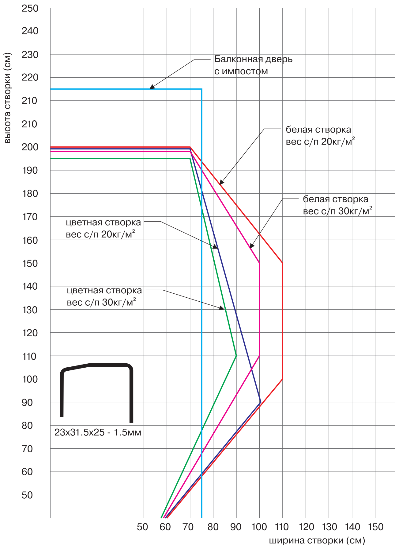
Диаграмма допустимых размеров поворотной (наклонно-поворотной) створки из профиля NOVOLINE COMFORT
