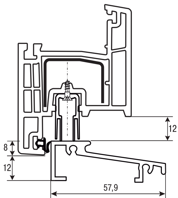
4.1 Система 5800 с холодным порогом
