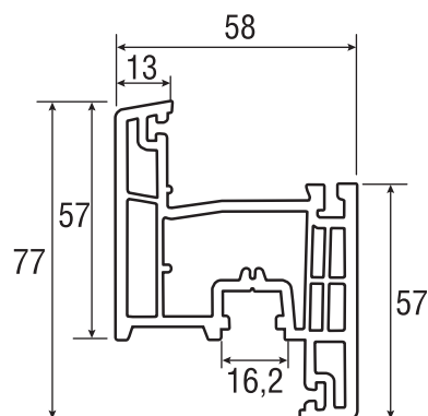
2.1.2 Профиль створки арт. 5821M4K
