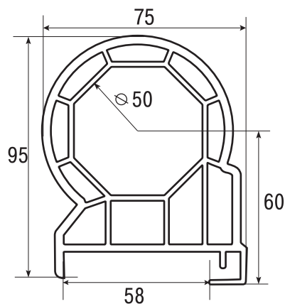
2.1.12 Профиль трубы для эркерных окон арт. НП 105
