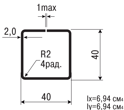
5.3 Армирующий профиль арт. 655 для арт 612, ДБ 355
