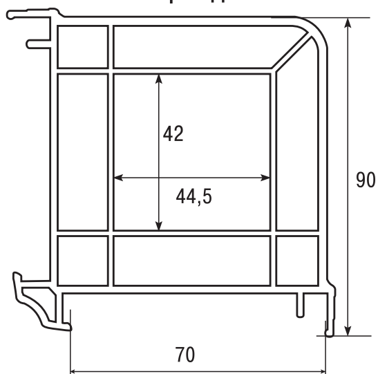
3.1.14 Соединитель угловой арт. БД 355
