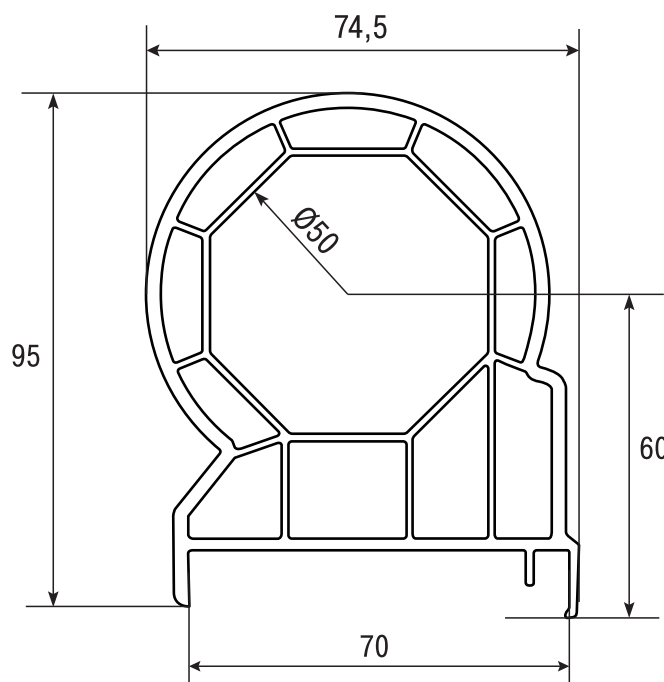
3.1.13 Труба с накладкой ПВХ для эркерных окон арт. БД 340
