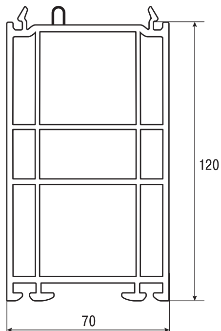
3.1.11 Профиль расширительный 120 мм арт. БД 363
