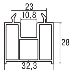
2.1.8 Профиль подставочный арт. 343 с пазом
