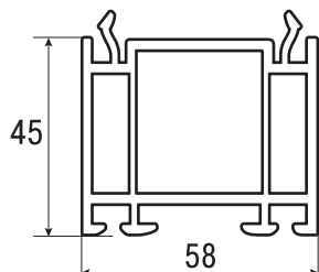
2.1.15 Расширитель 45 мм арт. БР 545
