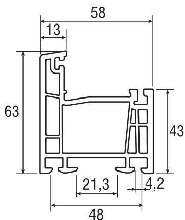
2.1.1 Профиль рамы арт. 5811M4K
