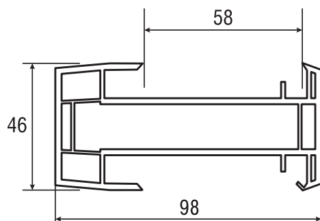
2.1.21 Заглушка для шульпа арт. K734
