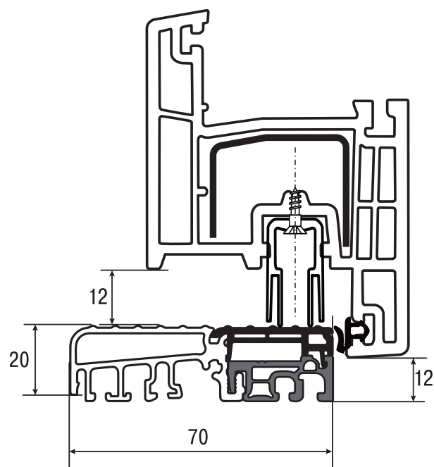
4.2 Система 5800 с теплым порогом
