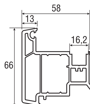
2.1.13 Профиль штульпа арт. 506
