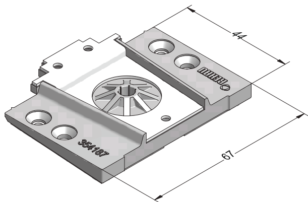
Механический соединитель импоста 78 и коробки, литой металлический
