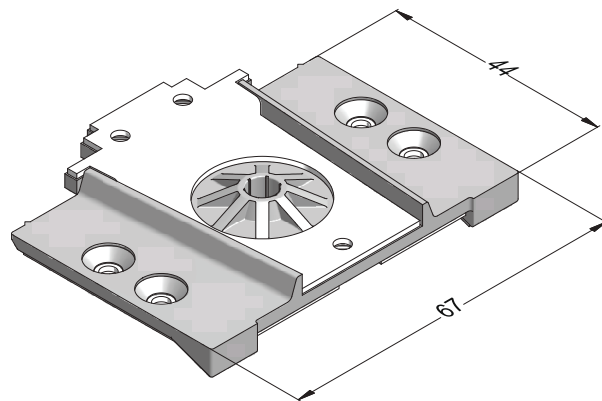
Механический соединитель импоста 78 и створки, литой металлический
