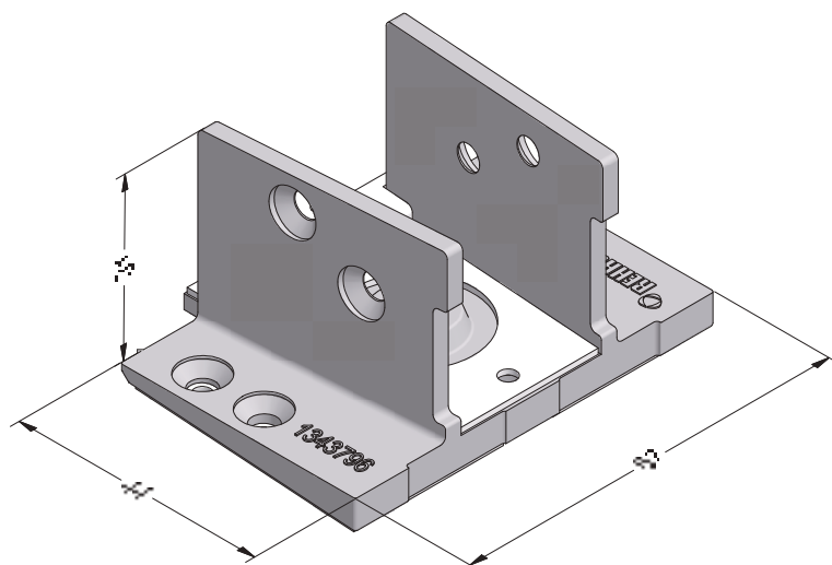
Механический соединитель импоста 78 и коробки, литой металлический
