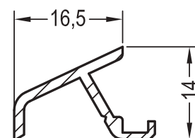
Слезник 14/70
