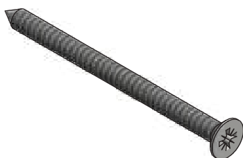
Шуруп 4,2 x 60 (ISO 7050), сталь оцинкованная
